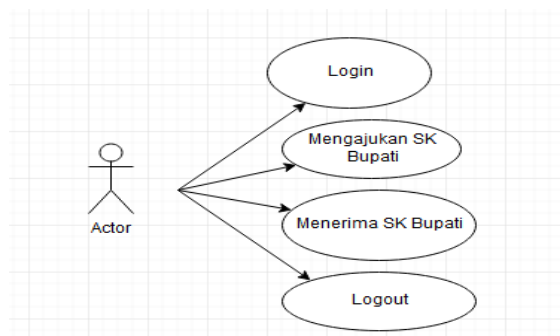
Gambar 3. Use Case Diagram Dinas Sistem Informasi Arsip Data Pengajuan SK Bupati
