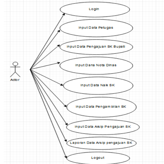
Gambar 4. Use Case Diagram Admin Perundang-undangan Sistem Informasi Arsip Data Pengajuan SK Bupati
