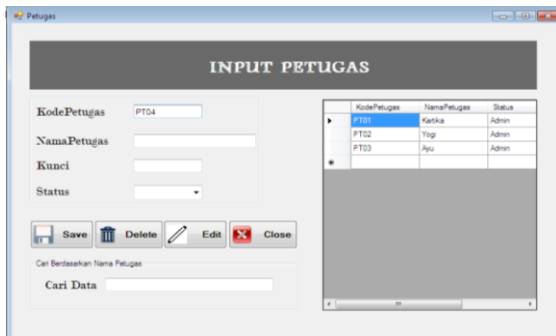
Gambar 9. Rancangan Dialog Input Data Petugas
